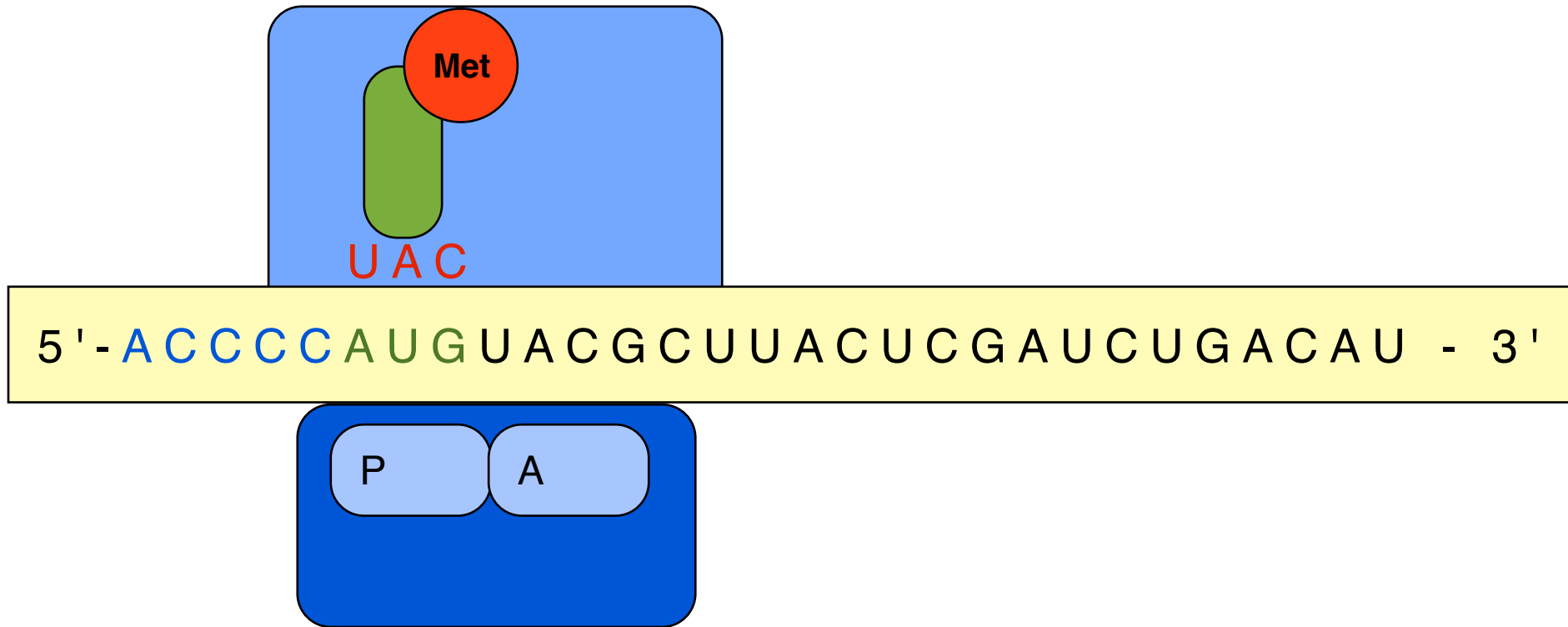
Funktionsbereites Ribosom
