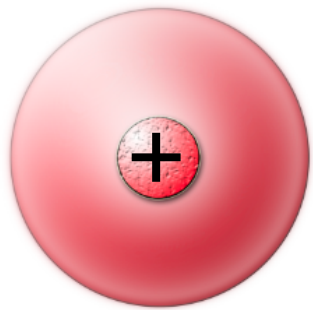
\text{H}^+ -Ion
